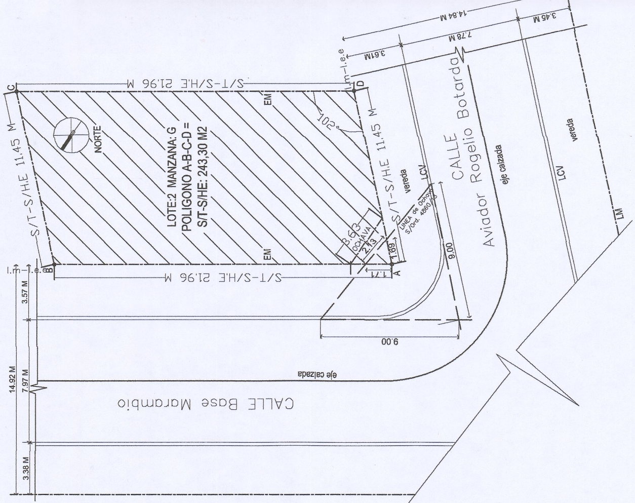
PLANIMETRIA esc: 1:250
