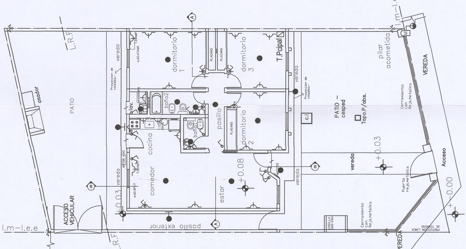
PLANTA RELEV. INSTALACION ELECTRICA
